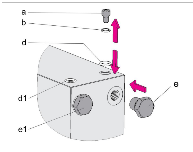
5. ábra: példa, vezeték nélküli hidraulikacsatlakozók előkészítése
