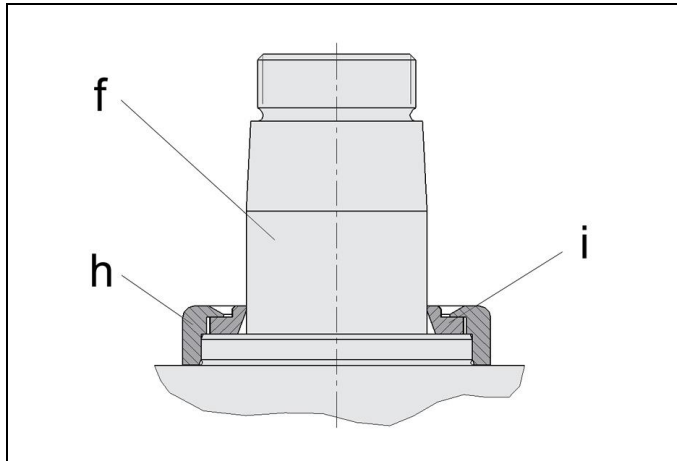
8. ábra: Fémházas porhúzó
