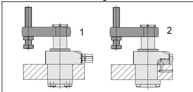
3. ábra: Összeszerelési lehetőségek
