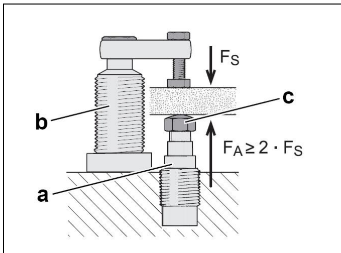
Fig. 2: Principio, trasferimento di forza all'irrigidimento
