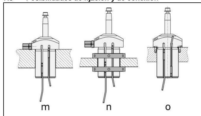
Fig. 3: Posibilidades de conexión
