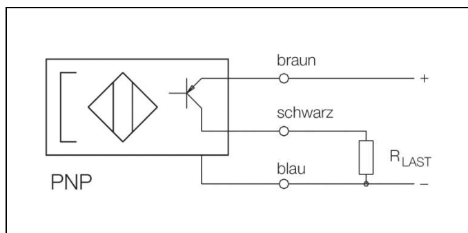
Fig. 9: Esquema eléctrico para PNP (+) sensor magnético
