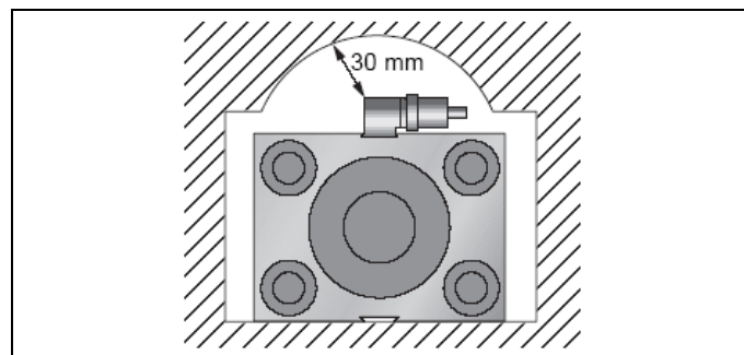
Fig. 10: Distancia mínima de los sensores a los protectores, etc.
