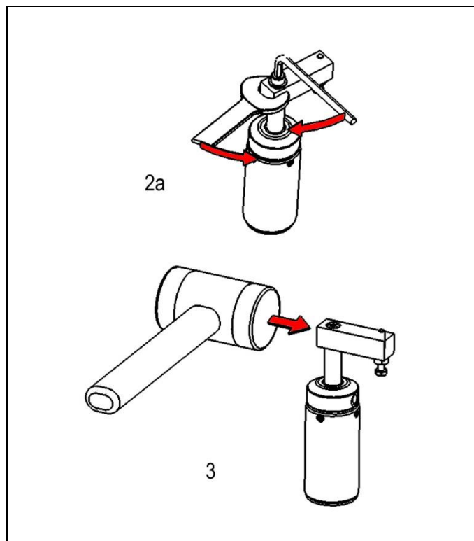
Fig. 5: Montaje / desmontaje - ejemplo
