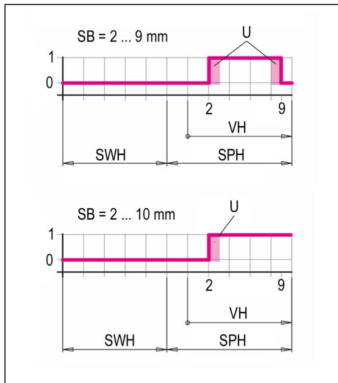
Fig. 12 : Courbe du signal
