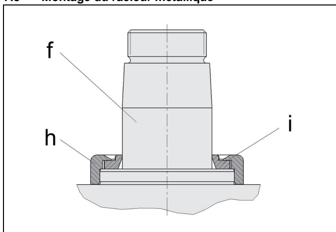
Fig. 9: Racleur métallique
