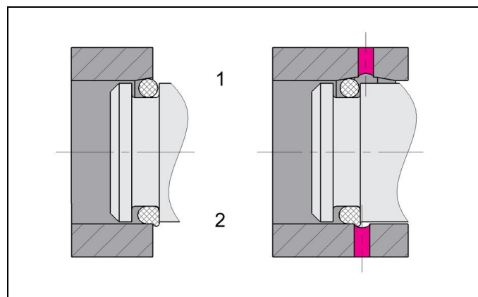
Fig. 6: Installation par chanfrein d'entrée et alésage transversal
