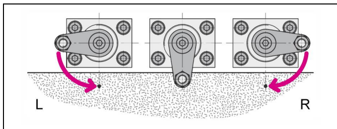
Fig. 3: Sens de pivotement (L = à gauche, R = à droite)
