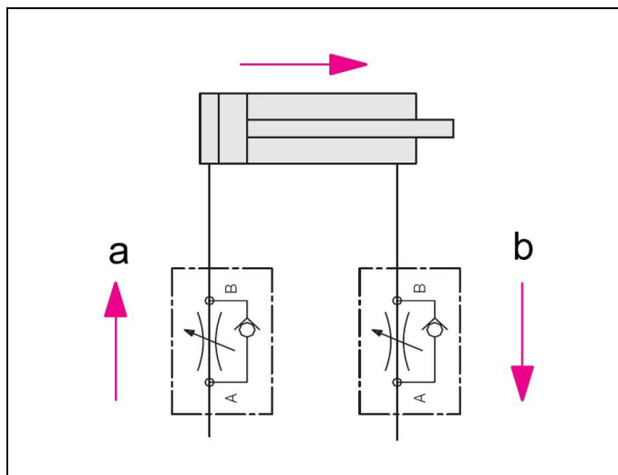
Fig. 2: Schéma hydraulique avec étrangleurs
