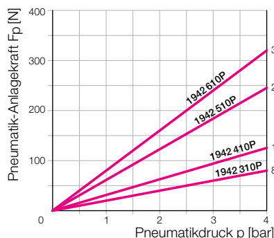
Pneumatik-Anlagekraft in Abhängigkeit vom Pneumatikdruck
