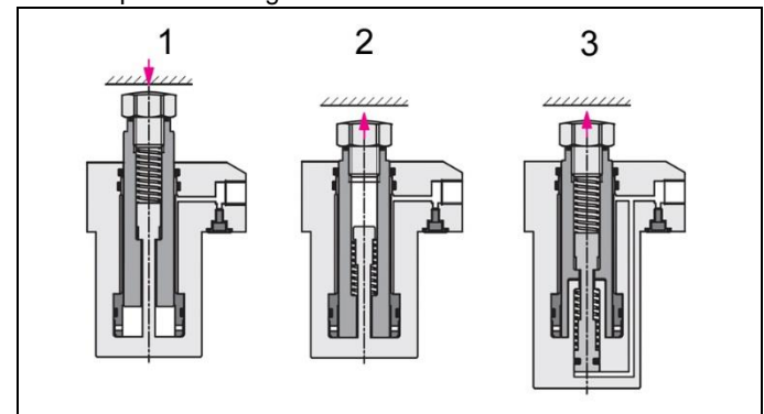
Fig. 2: 1-Forza della molla/ 2-Pressione pneumatica/ 3- Pressione idraulica con forza della molla
