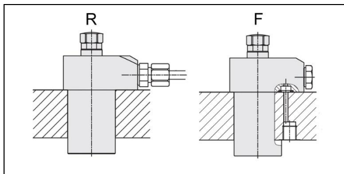
Fig. 3: R-Collegamento con raccordi / F-Collegamento con flangia
