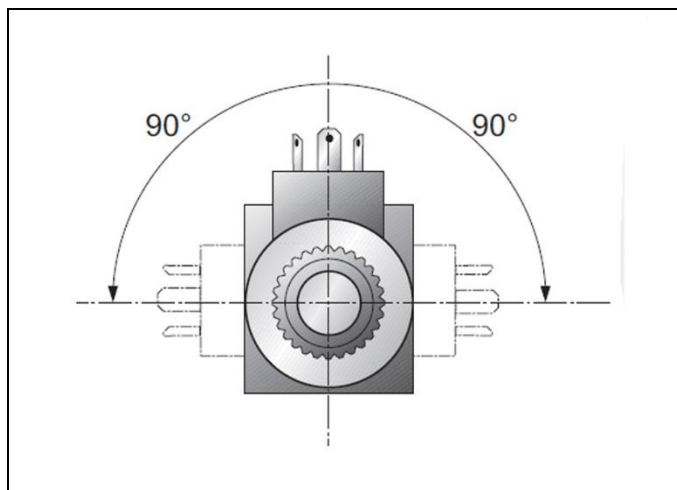
Fig. 2 : Bobines d'électro-aimant
