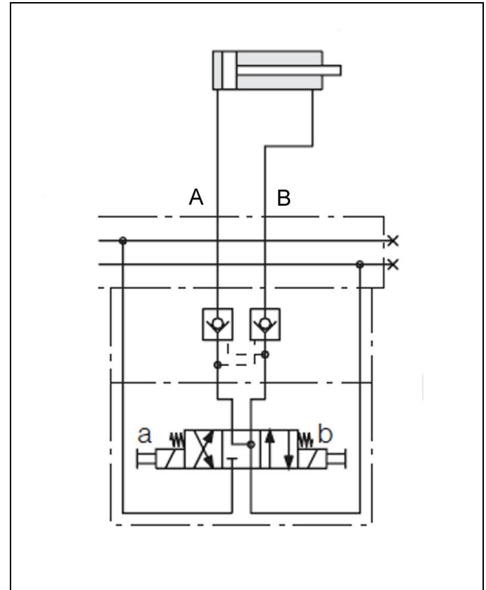
Fig. 6 : Représentation sur le schéma hydraulique
