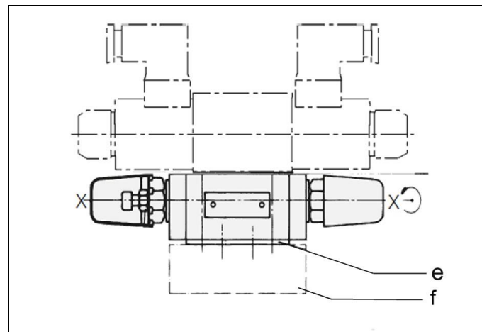
Fig. 3 : Étrangleur double unidirectionnel
