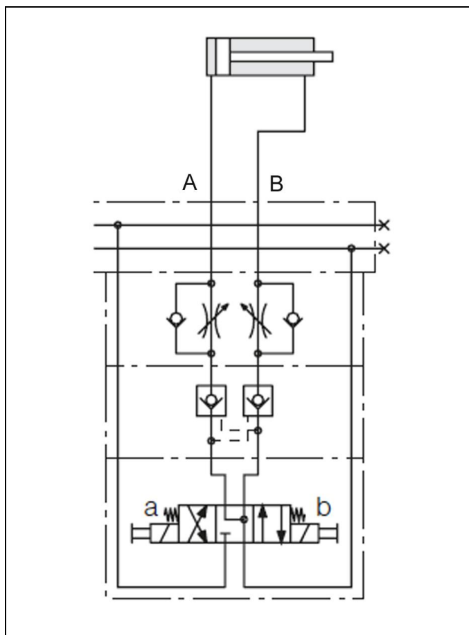
Fig. 7 : Représentation sur le schéma hydraulique
