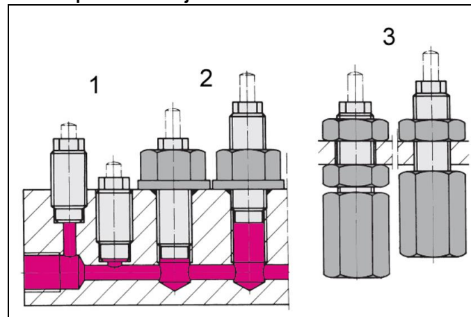
Fig. 2: Posibilidades de fijación
