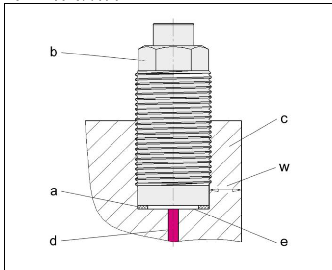
Fig. 3: Instalación de la junta axial en la superficie plana
