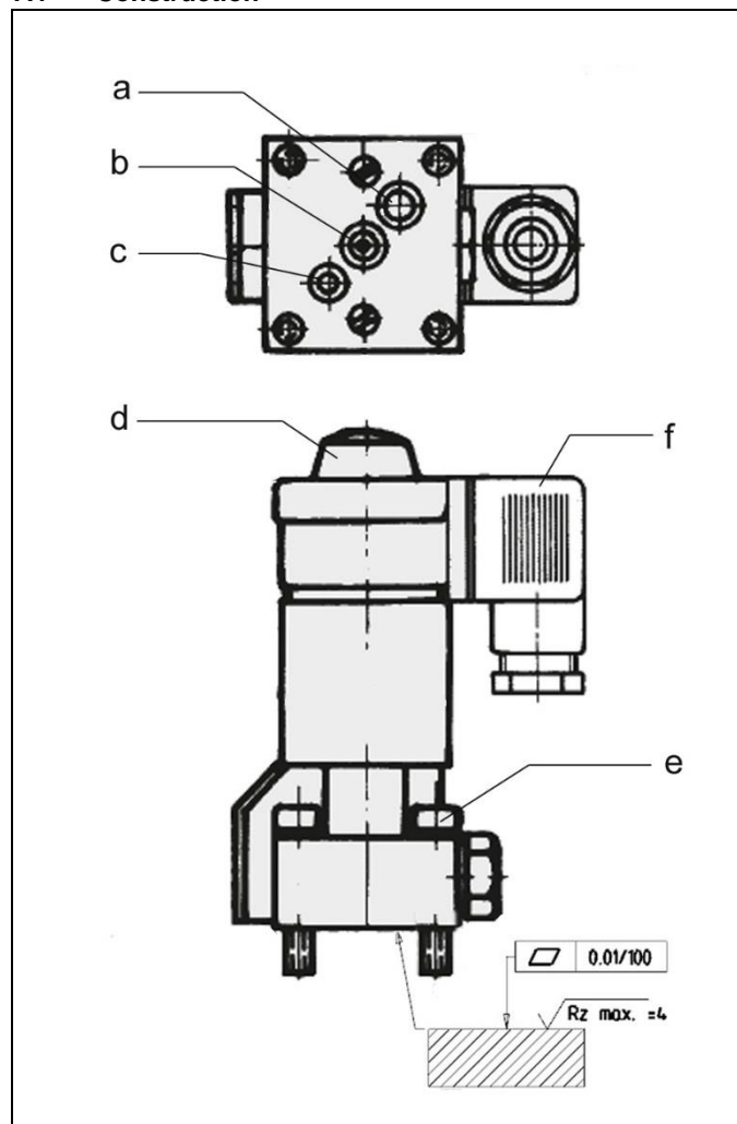
Fig. 1 : Construction des valves 2/2 et 3/2
