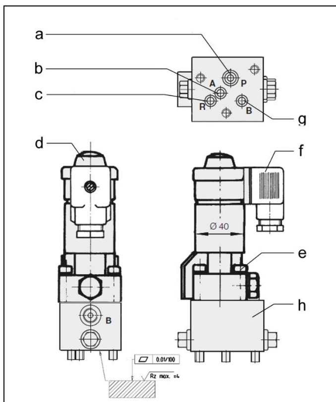
Fig. 2 : Construction de la valve 4/2
