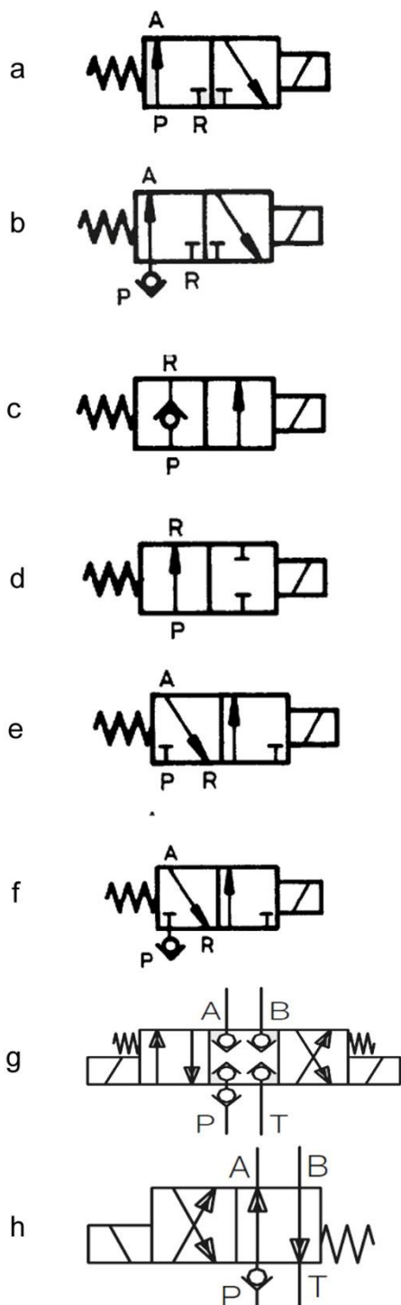
Fig. 4 : Représentation sur le schéma hydraulique
