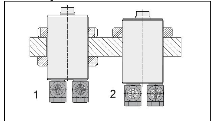
Abb. 2: Befestigungsmöglichkeiten
