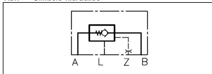
Fig. 3: Representación en el esquema hidráulico
