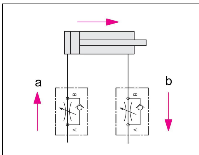
Fig. 2: Schéma hydraulique avec éjecteurs
