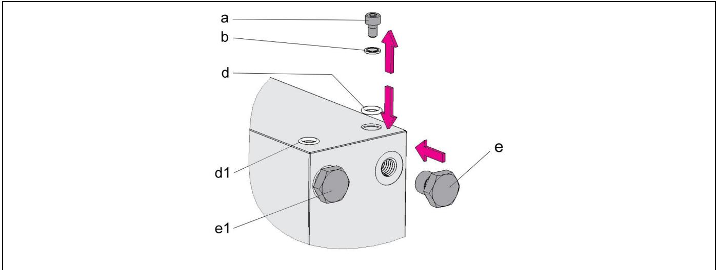
Abb. 3: Beispiel, Vorbereitung für leitungslose Hydraulikanschlüsse
