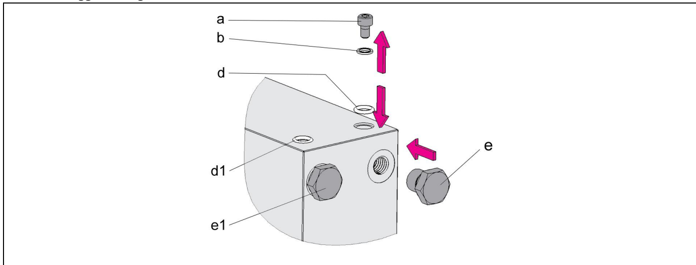
Fig. 3: Esempio, installazione della versione a flangia (senza tubi)
