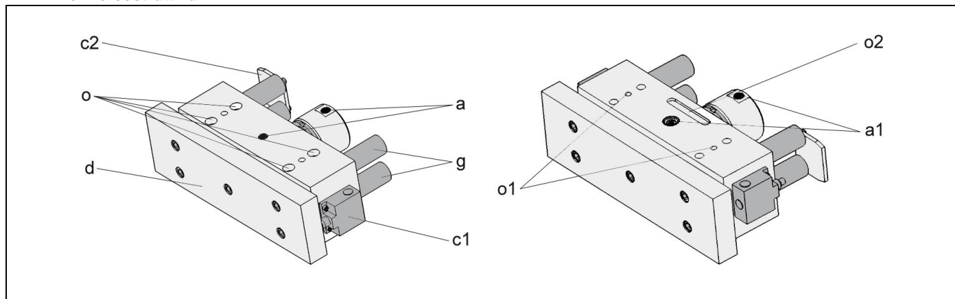
Fig. 1: Componenti, opzionalmente con due finecorsa meccanici
