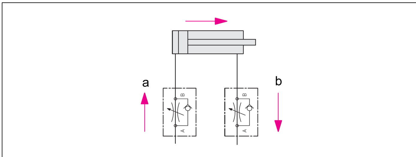
Fig. 2: Schema idraulico con valvole di ritenuta e strozzamento
