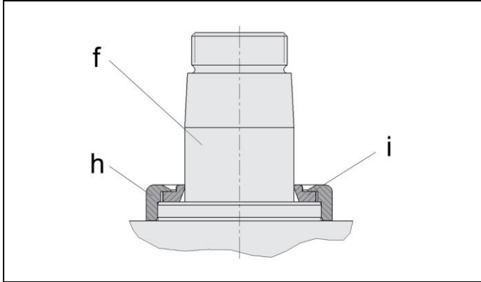
Abb. 8: Metallabstreifer
