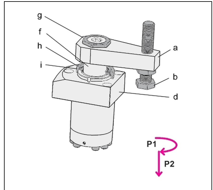
Abb. 1: Komponenten
