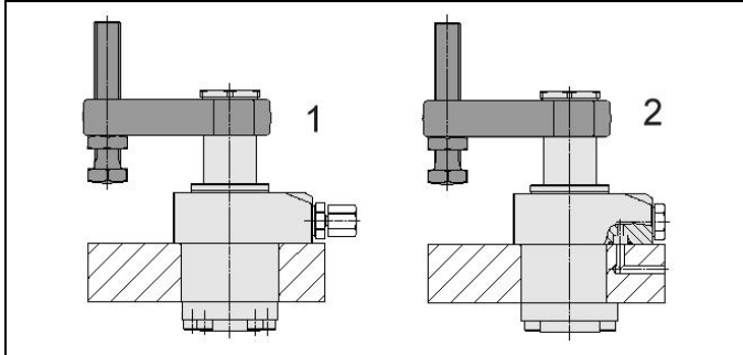
Abb. 3: Montagearten
