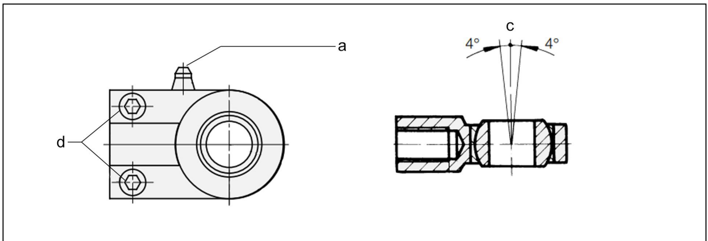
Abb. 2: Gelenkkopf
