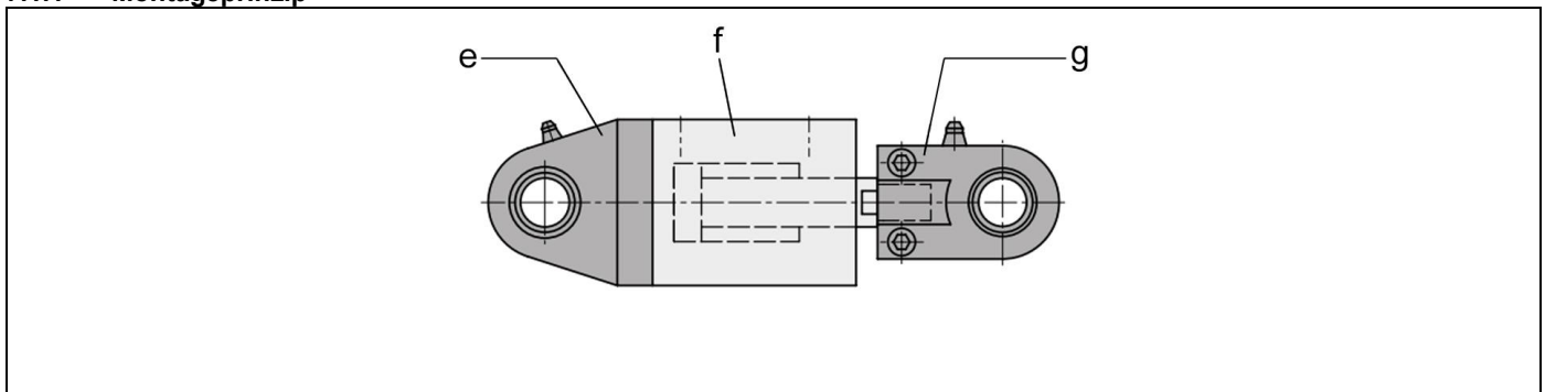
Abb. 3: Montage Beispiel
