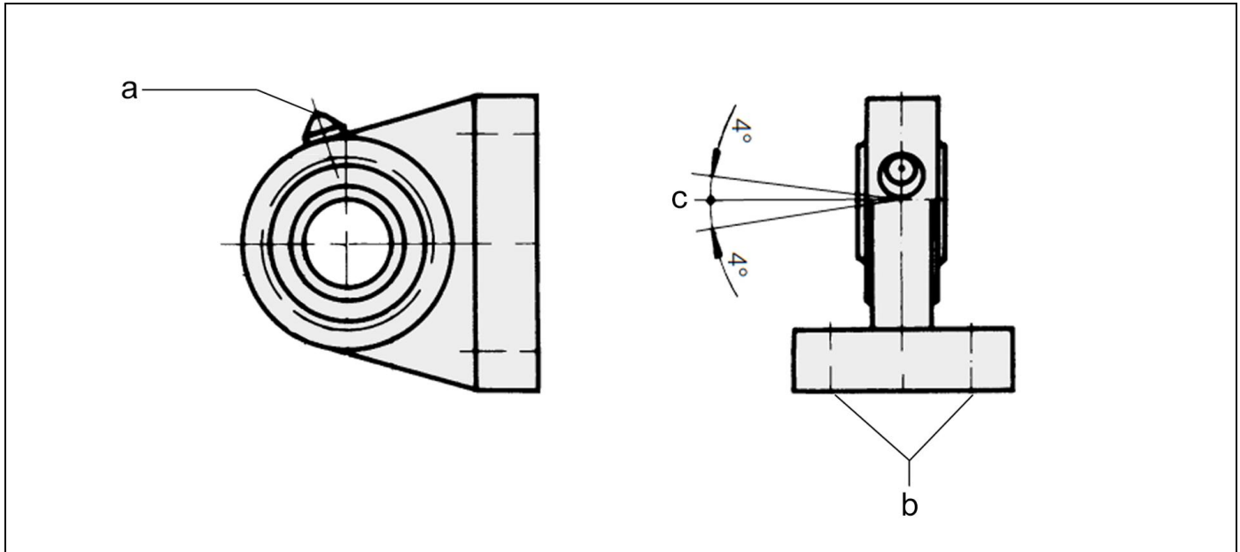
Abb. 1: Lagerbock
