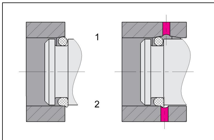
Abb. 4: Einbau über Einführungsfasen und Querbohrung
