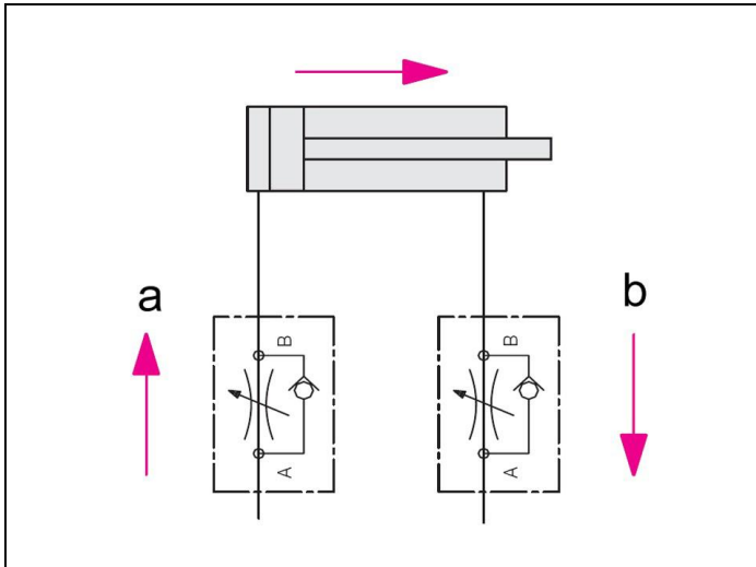
Abb. 2: Hydraulikplan mit Drosselrückschlagventilen
