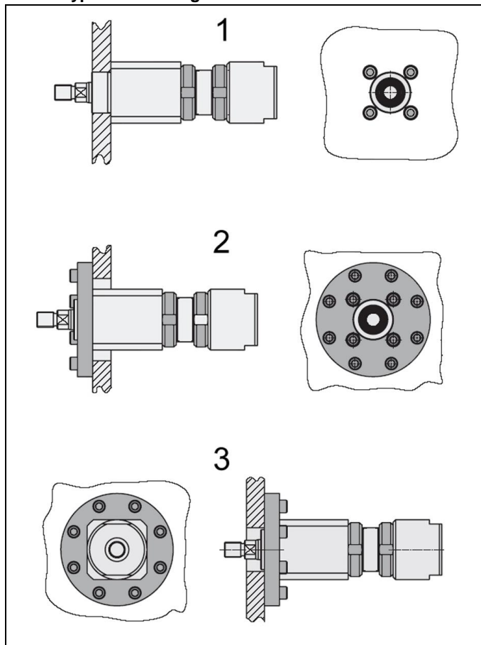
Fig. 2: Possibilités de fixation
