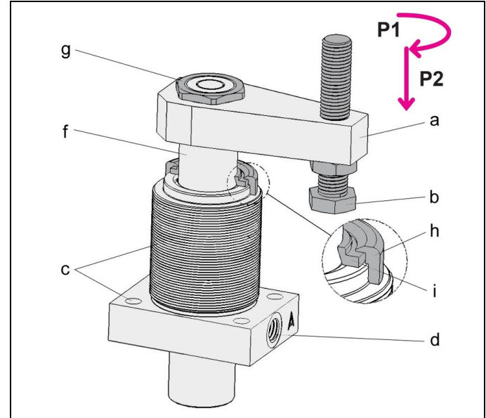
Fig. 1 : Composants
