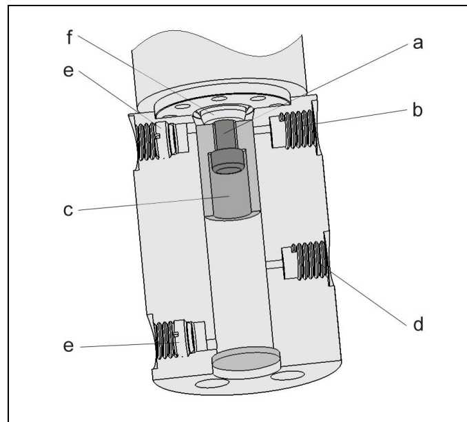
Fig. 13 : Construction
