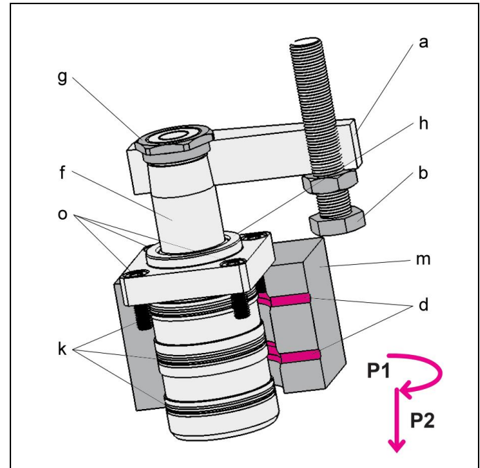
Fig. 1 : Composants
