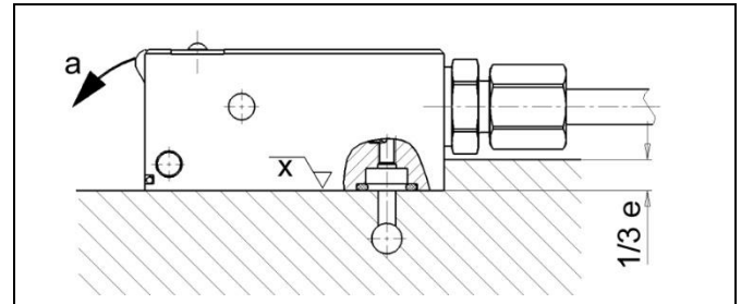
Abb. 2: Tiefspann- Blockzylinder abgestützt (Befestigung und Unterstützung 1/3 * e)
