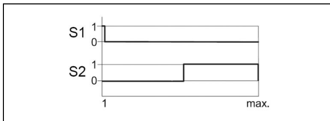
Fig. 11: Courbe du signal pendant le procédé de bridage
