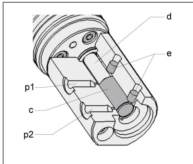
Fig. 13 : Construction
