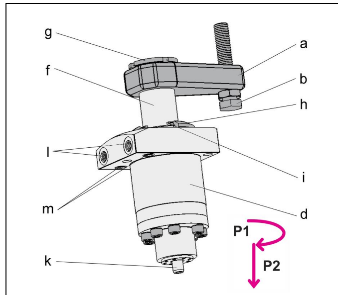
Fig. 1 : Composants
