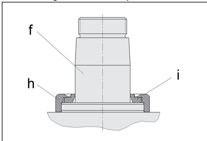
Fig. 8: Racleur métallique
