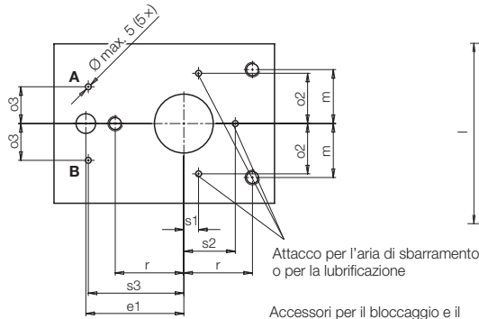
Schema dei collegamenti
