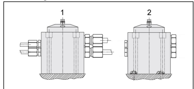
Abb. 2: Befestigungsmöglichkeiten
