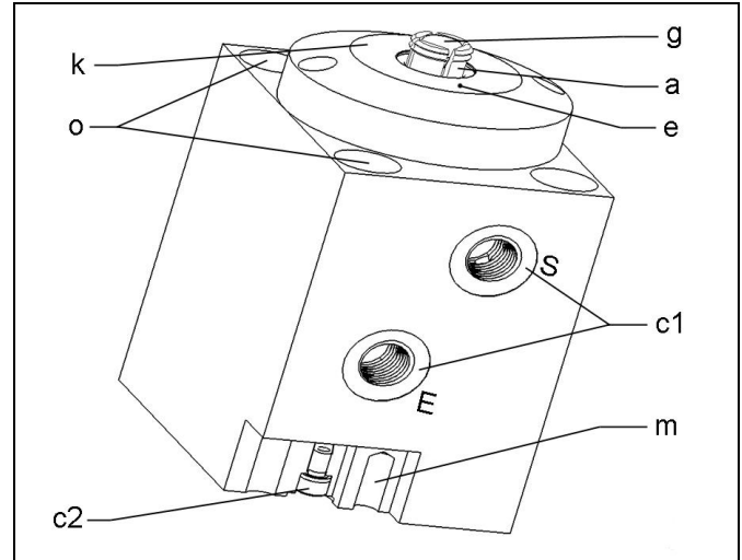
Abb. 1: Komponenten
