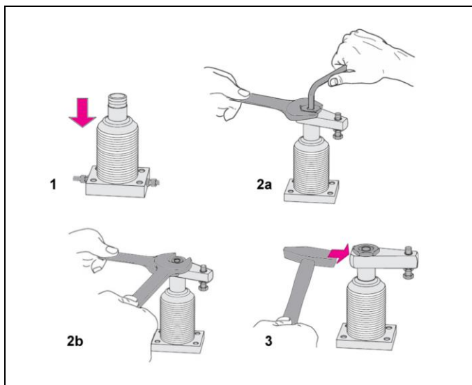
Fig. 8: Montage / démontage - exemple
