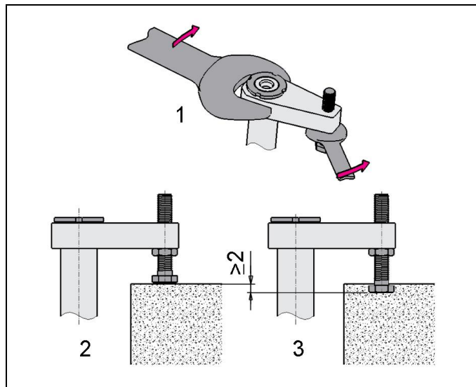
Fig. 9: Exemple du réglage de la vis de pression
