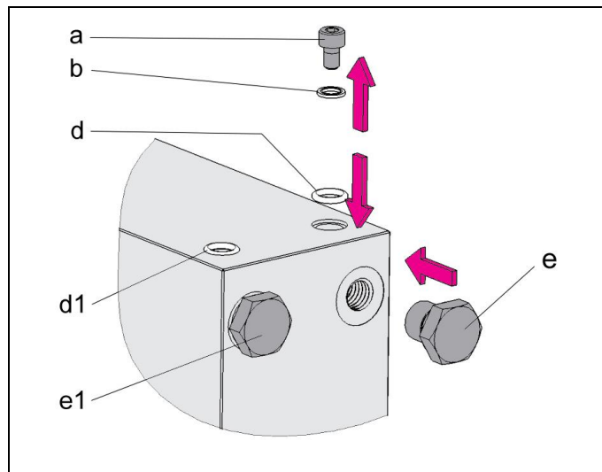
Fig. 7 : Exemple, préparation pour des connexions hydrauliques sans tuyauterie
