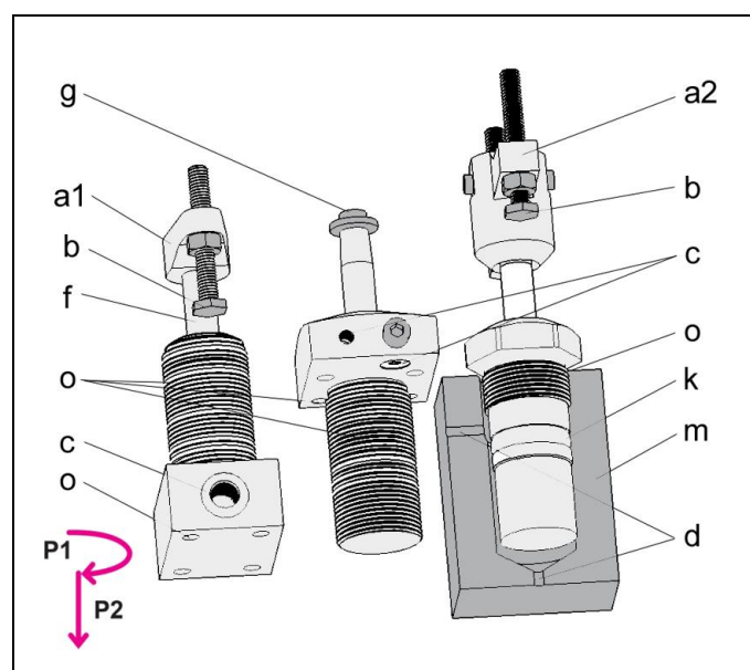
Fig. 1 : Composants
