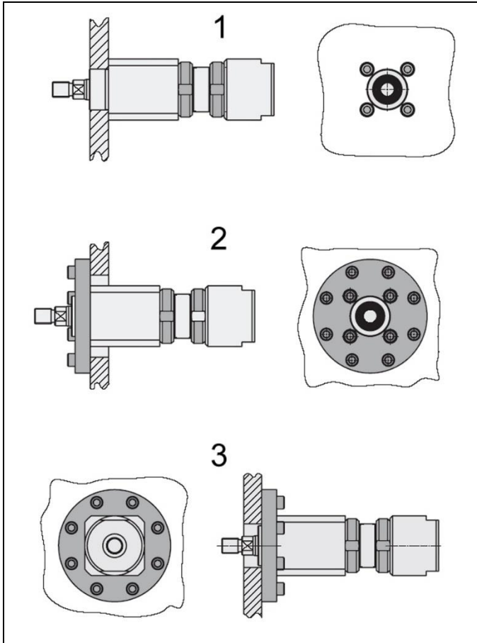
Fig. 2: Possibilità di fissaggio
