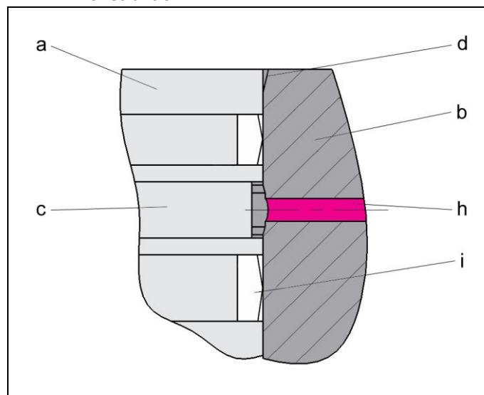
Bild 4: Komponenter
