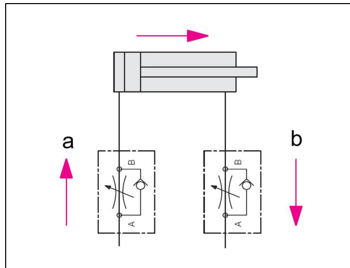
Bild 3: Hydraulikschema med strypbackventiler
