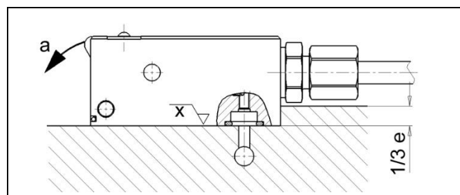
Fig. 2: Cilindro bloque de sujeción inclinado soportado (accesorio y soporte 1/3 * e)
