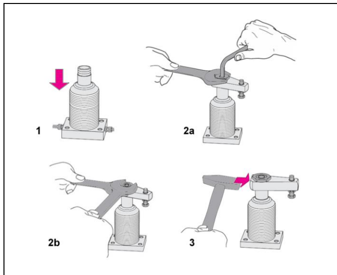
Fig. 7: Montaje / desmontaje - ejemplo
