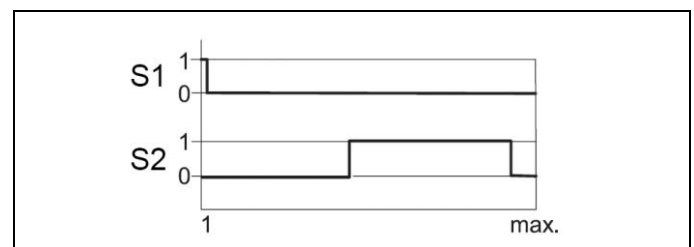
Abb. 13: Signalverlauf Entspannvorgang
