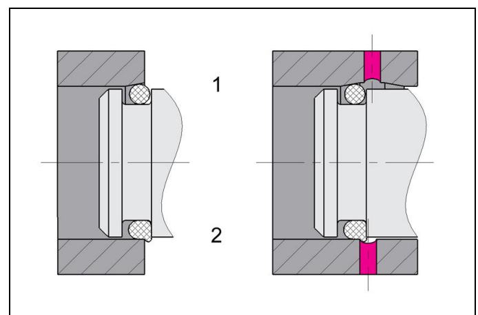
Abb. 5: Einbau über Einführungsfasse und Querbohrung
