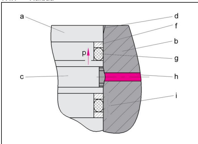
Abb. 4: Komponenten
