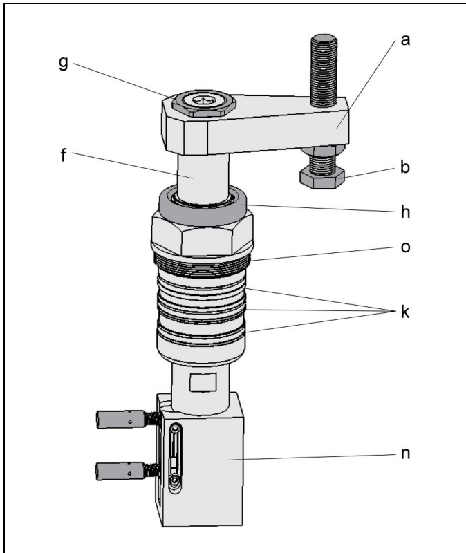
Abb. 1: Komponenten
