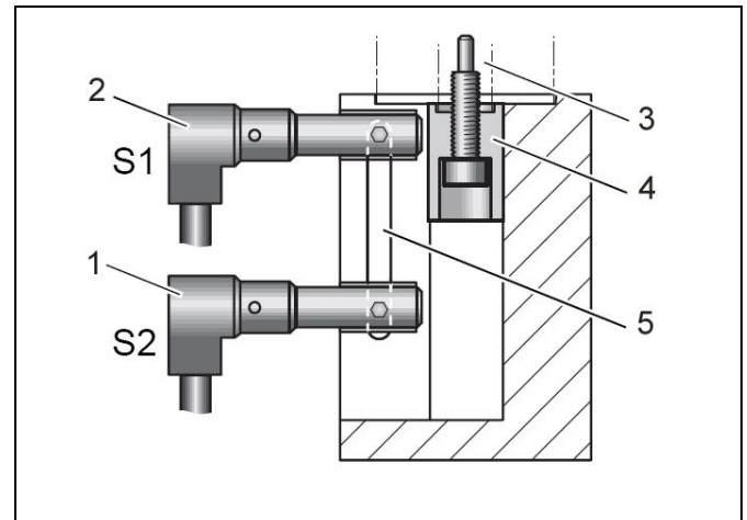
Abb. 11: Aufbau der elektrischen Positionskontrolle
