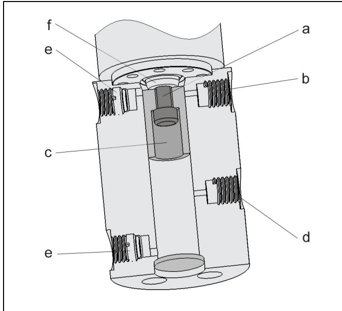
Abb. 10: Aufbau
