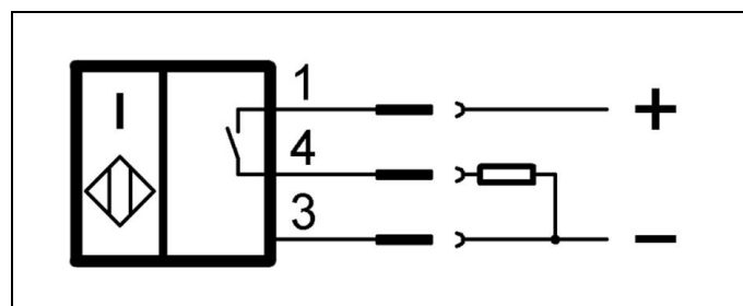
Fig. 11 : Schéma pour pnp (+) capteur inductif
