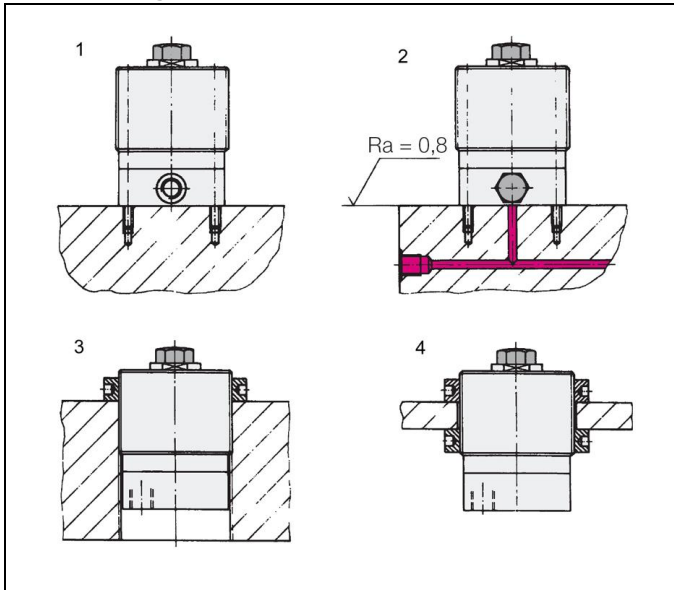
Abb. 2: Befestigungsmöglichkeiten
