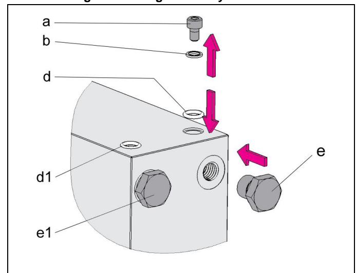
Abb. 5: Beispiel, Vorbereitung für leitungslose Hydraulikanlüsse
