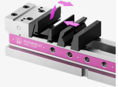
QIS-Wechselbacke bis Nutende hochschieben und abklicken
