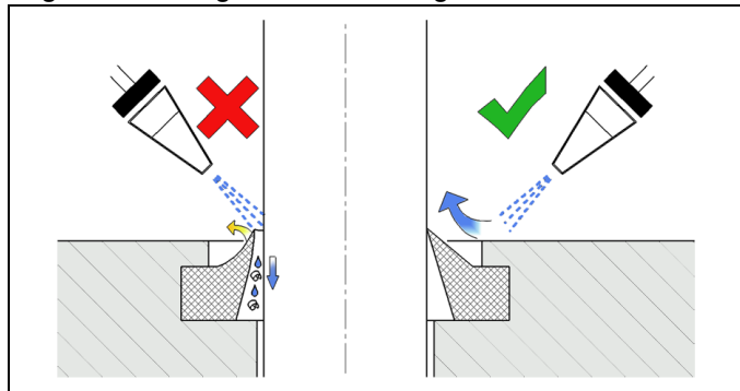
Fig. 5: Introduzione di trucioli tramite getto diretto di lubrorefrigerante
