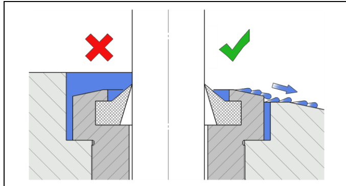
Fig. 6: Deflusso del lubrorefrigerante, sull'esempio di un elemento filettato
