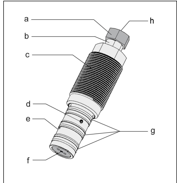
Abb. 1: Komponenten
