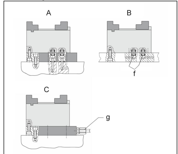
Abb. 2: Montagearten
