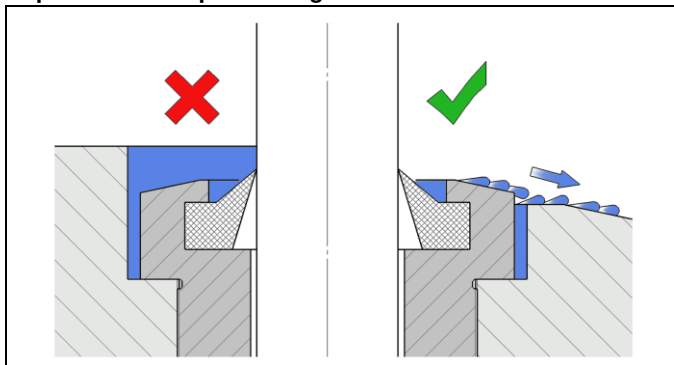
Fig. 6: Desagüe del líquido refrigerador, utilizando el ejemplo de un elemento enroscable
