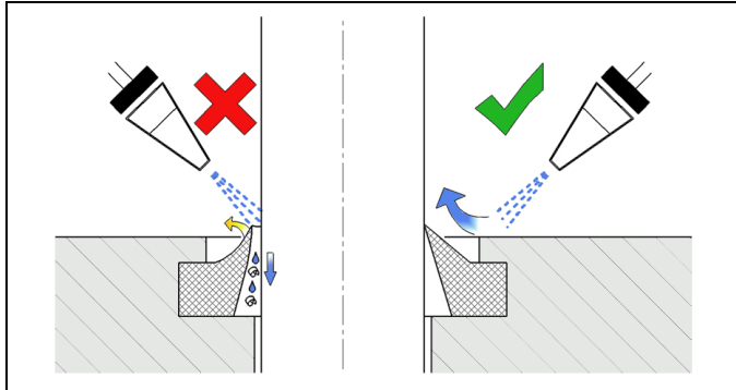
Fig. 5: Entrada de virutas por chorro directo de líquido refrigerador
