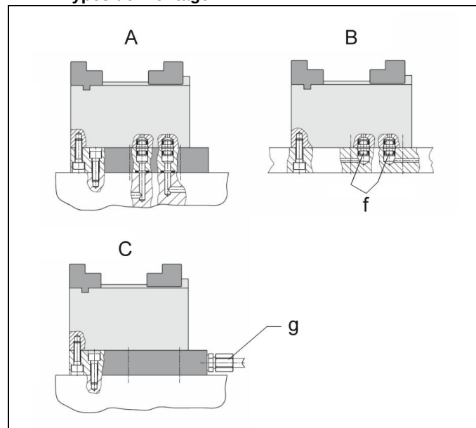
Fig. 2 : Types de montage
