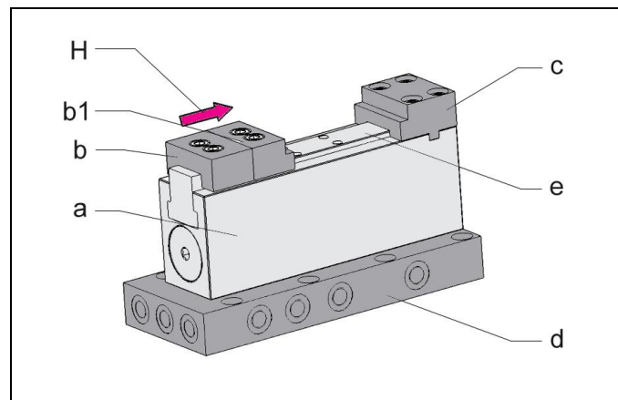
Fig. 1 : Composants
