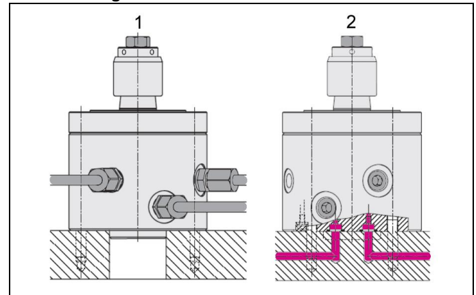
Abb. 2: Befestigungsmöglichkeiten
