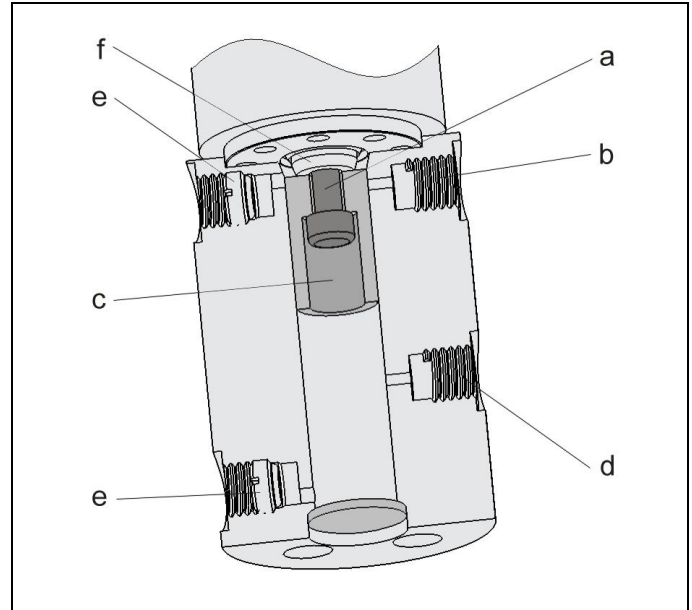
Abb. 13: Aufbau
