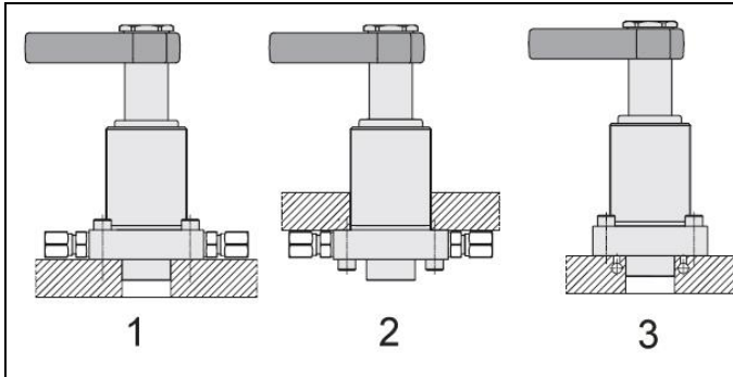
Abb. 3: Montagearten
