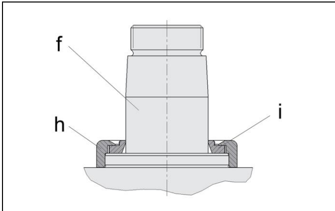
Abb. 8: Metallabstreifer
